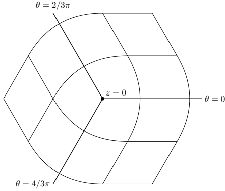
図 6: \omega = z^{-1}dz^4 のときの \mathcal{F}_\omega
