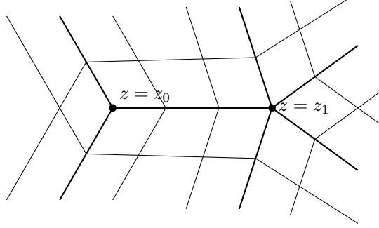
図 7: \omega = \frac{z-z_1}{z-z_0}dz^4 のときの \mathcal{F}_\omega .
