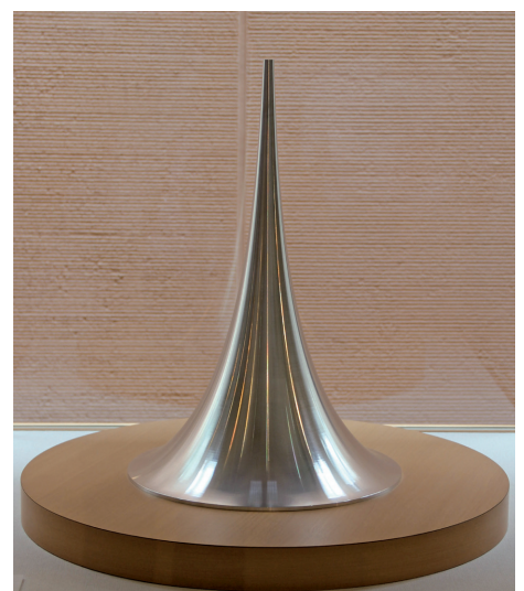
擬球 - 負の定曲率曲面 (ヤマダ精機制作、東大数学同窓会寄贈)
