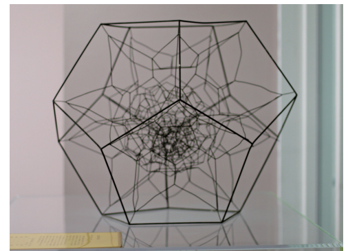
4次元空間内の正120胞体の模型
