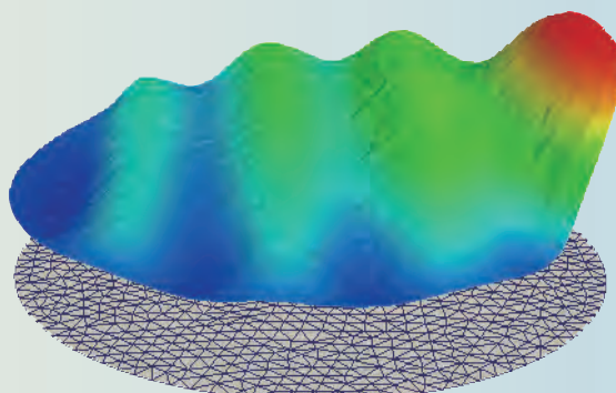
有限要素法による Poisson 方程式の数値解
